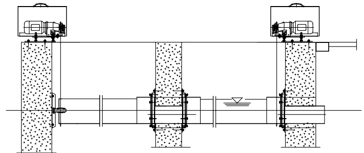
Motormanövrerad dekanteringsränna
