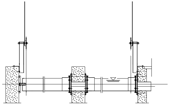
Handmanövrerad dekanteringsränna
